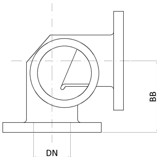
TIPO "A" (CON BRIDAS)
