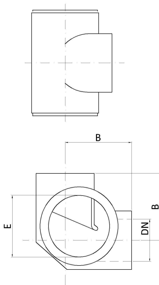
TIPO "B" (ROSCADOS)
